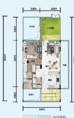
—— 首层平面分布图 ——
